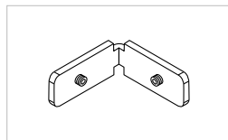
Esquadro para PT P003, PT P021, PT P022 e para perfil de reforço PT P015
